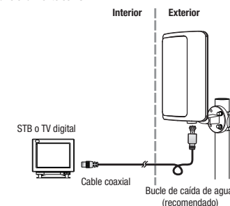
Fig. 3: Funcionamiento con STB
