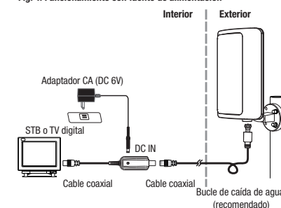
Fig. 4: Funcionamiento con fuente de alimentación
